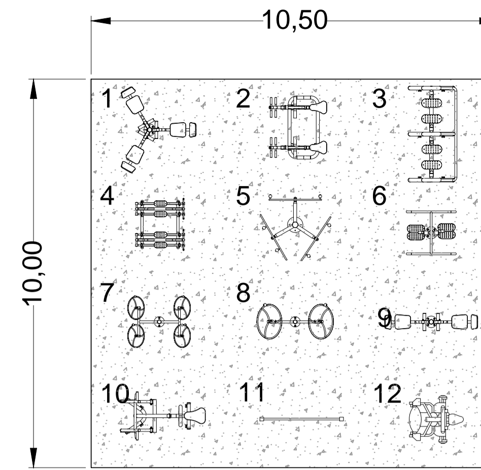
Detalhe da Implantação 1:100
