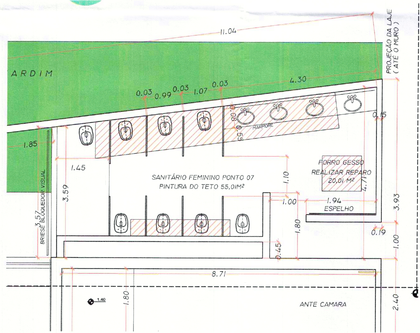
BANHEIROS FEMININOS DETALHES FORRO GESSO
