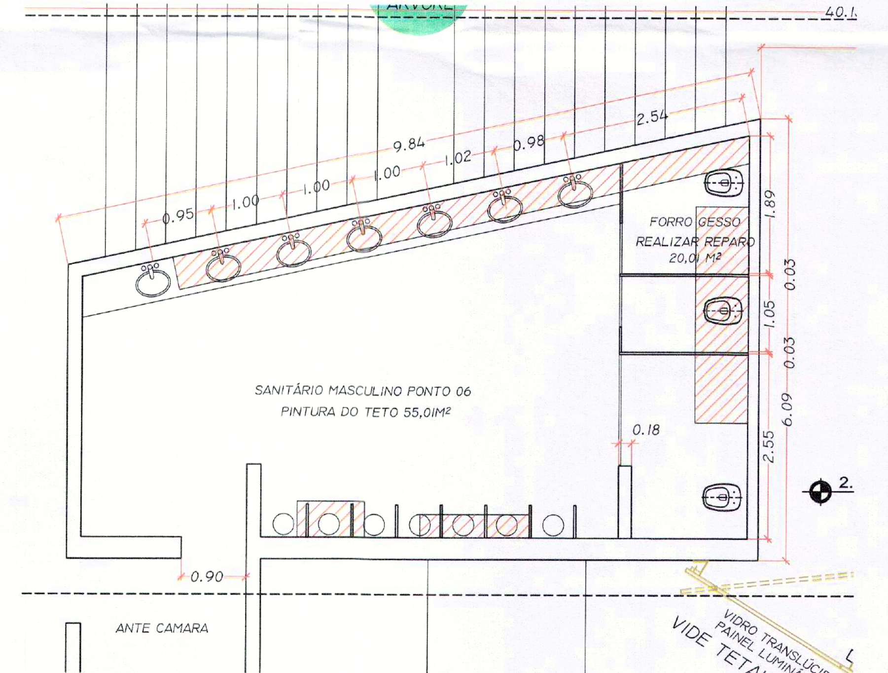
BANHEIROS MASCULINO DETALHES FORRO GESSO
