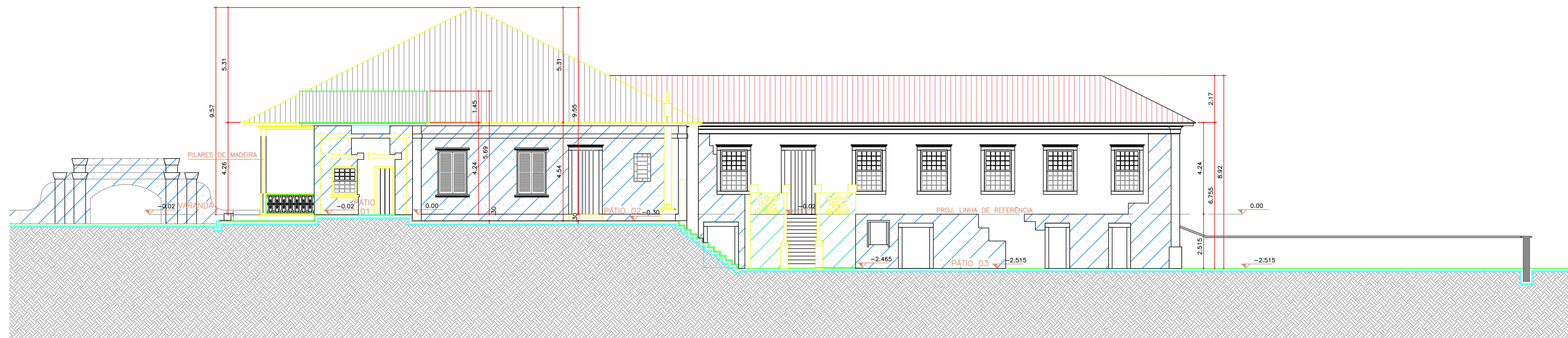
1 ELEVÇÃO 04 – LONGITUDINAL DIREITA ESC. 1:100
