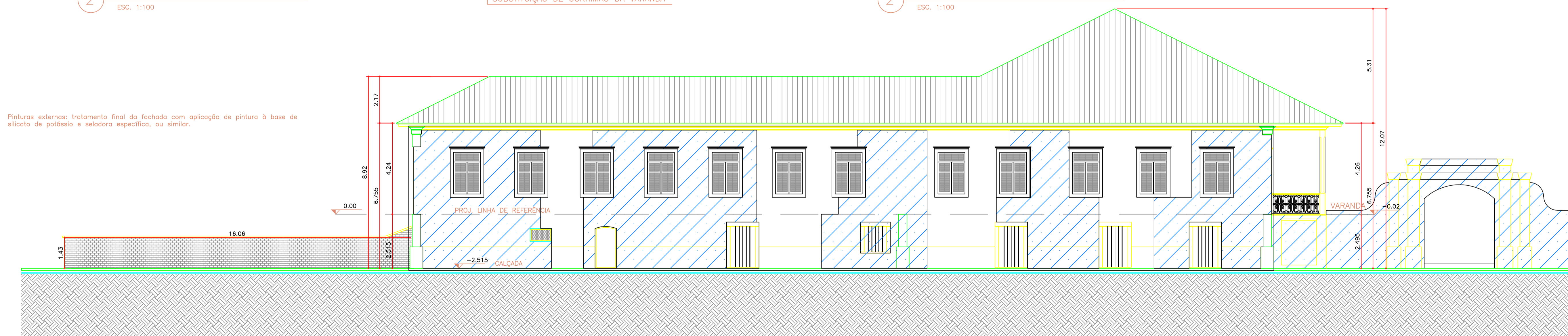
1 ELEVÇÃO 01 – LONGITUDINAL ESQUERDA ESC. 1:100
