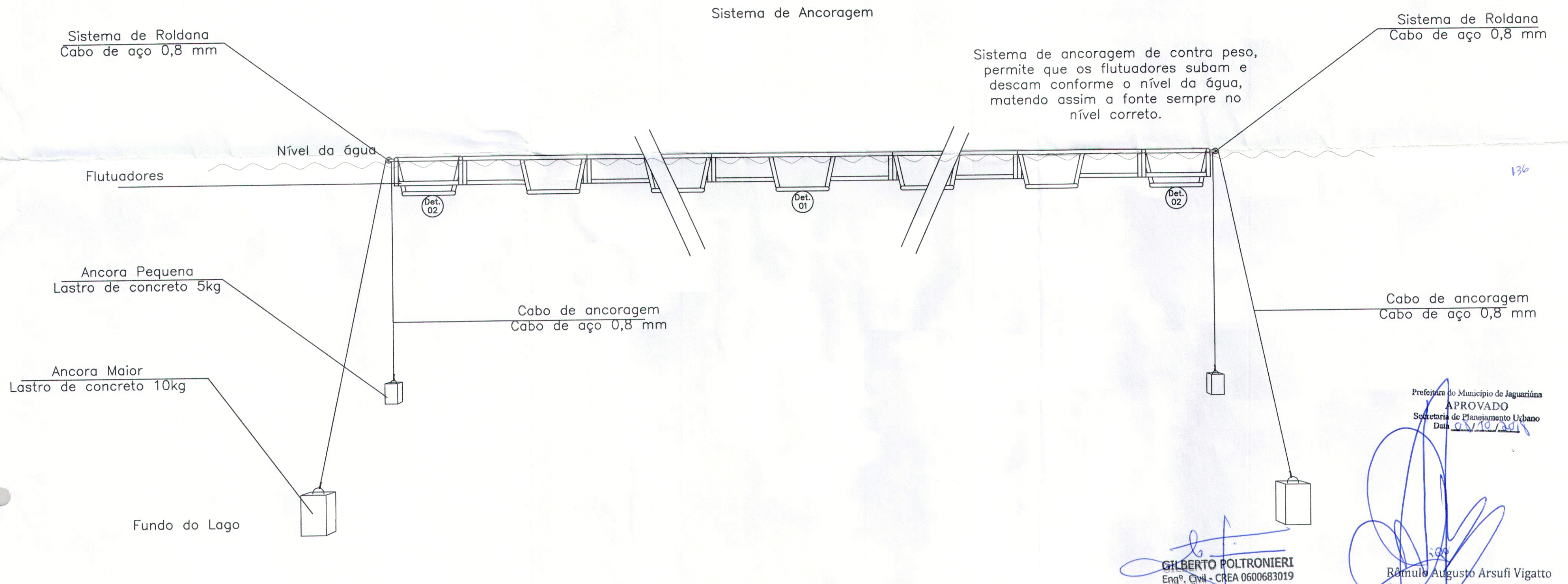
Det. 06 Sistema de Ancoragem
