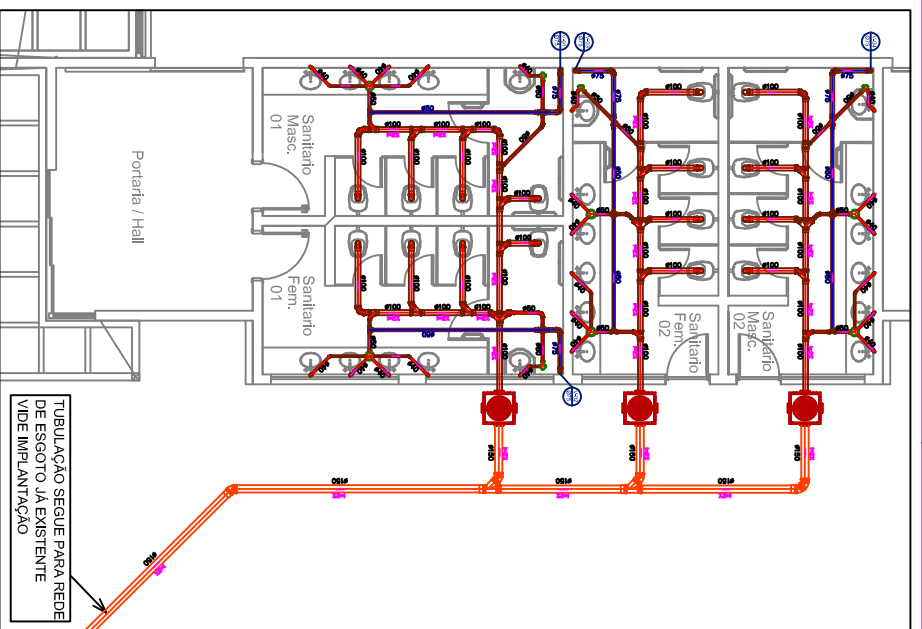
PLANTA BAIXA - DOS SANITÁRIOS - AUDITORIO ESC. 1:30
