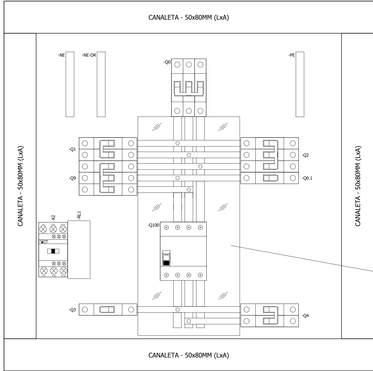
VISTA FRONTAL - PLACA DE MONTAGEM
