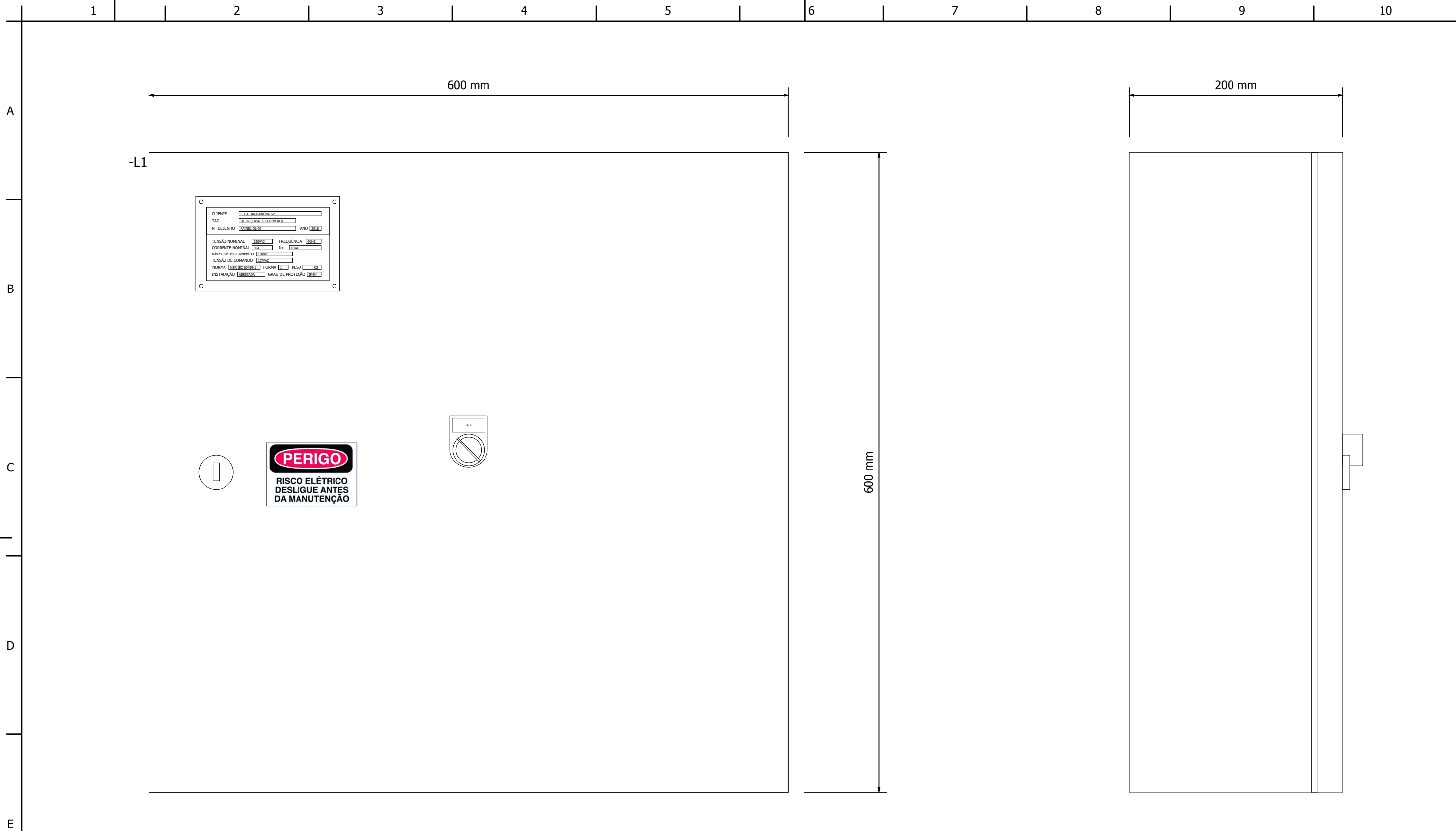
VISTA FRONTAL - PORTA
