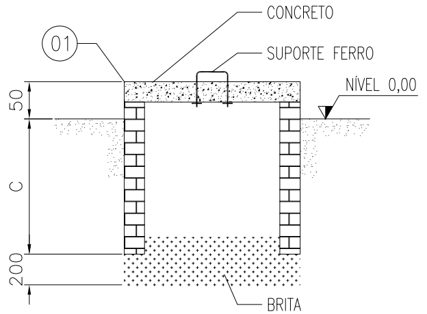
CORTE A-A
