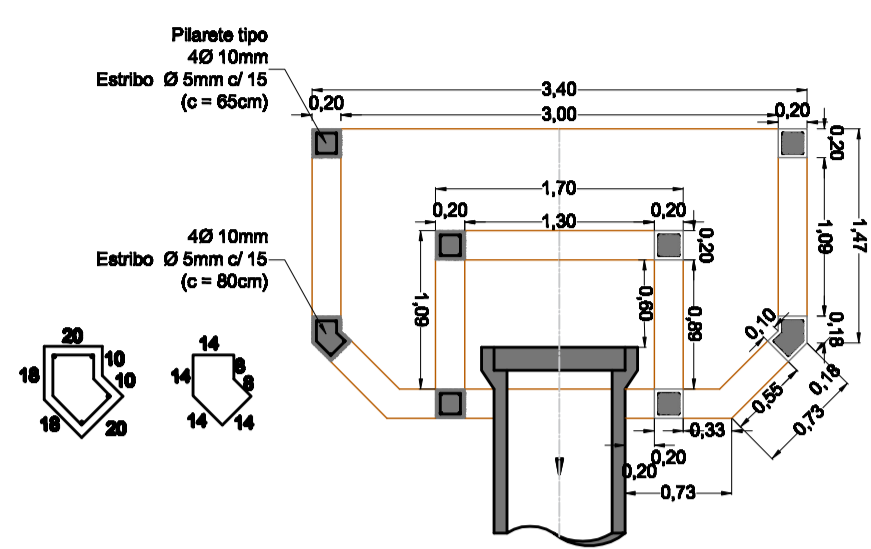
Planta Baixa 1:5
