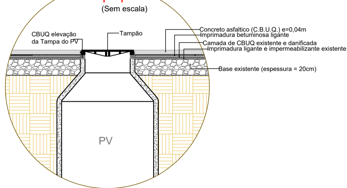
Detalhe asfalto próximo aos PVs. Serviço a ser executado pela Contratada, com equipe e materiais próprios
