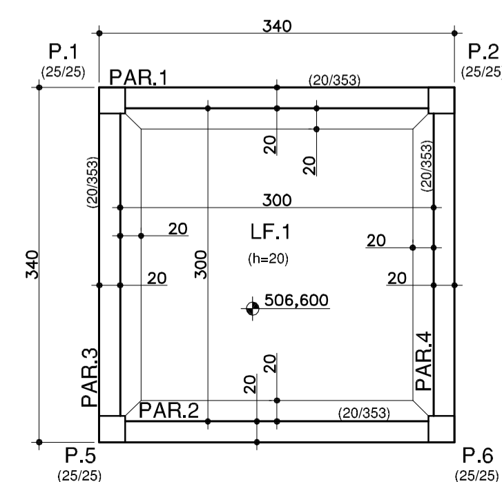
FORMA - PLANTA NÍVEL 506,600 FUNDO RESERVATÓRIO ESC. 1:50
