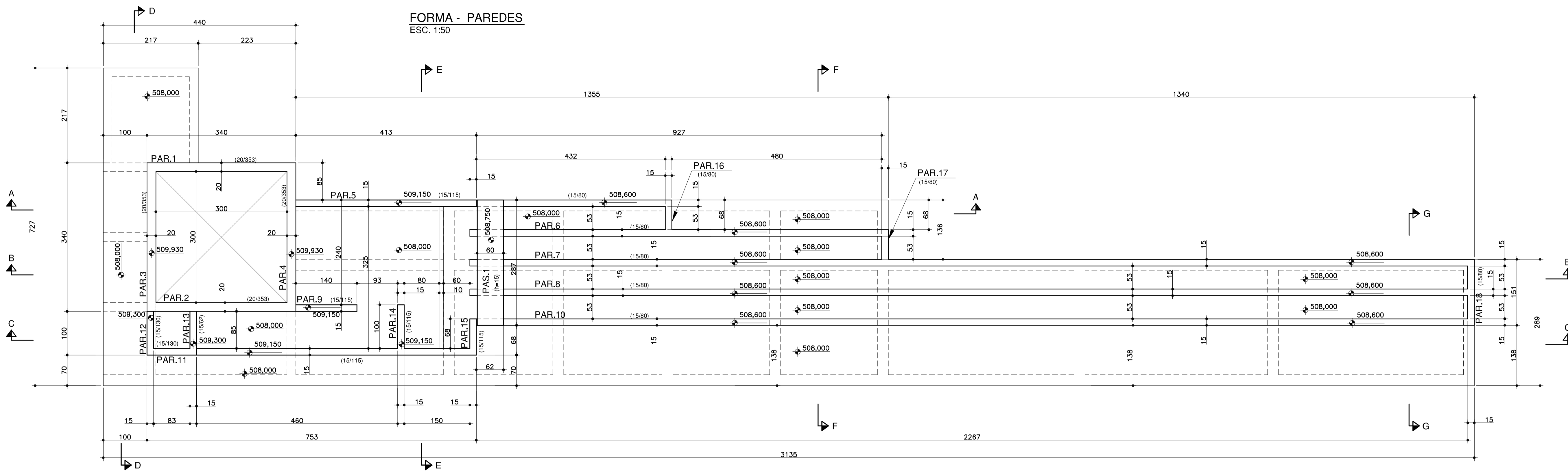
FORMA - PLANTA NÍVEL 508,000 ESC. 1:50
