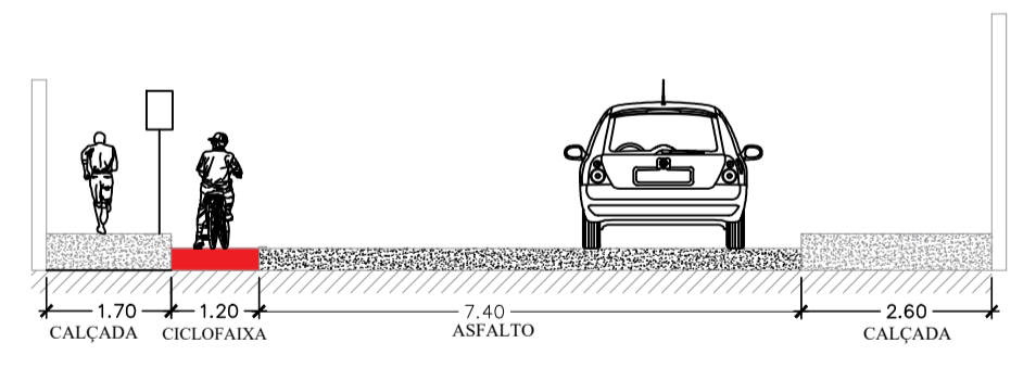
DET. 01
