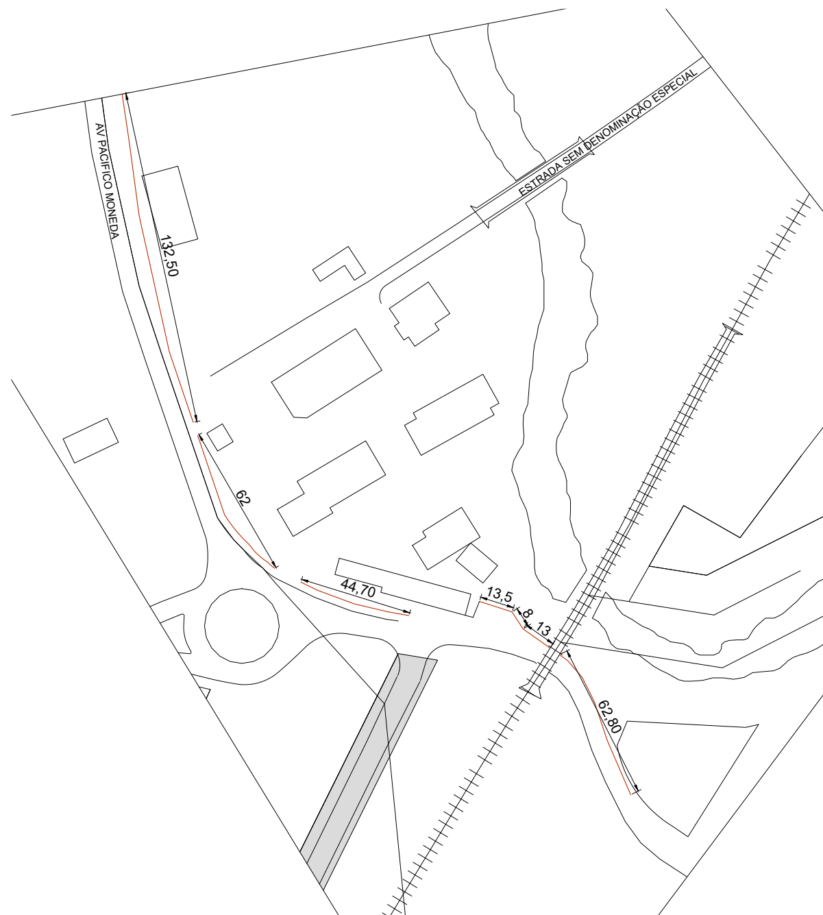
PLANTA BAIXA OBRAS sem escala
