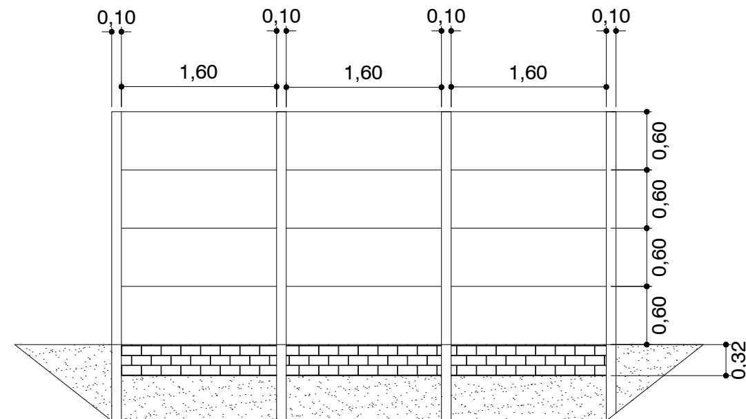
Vista frontal - muro do obras sem escala
