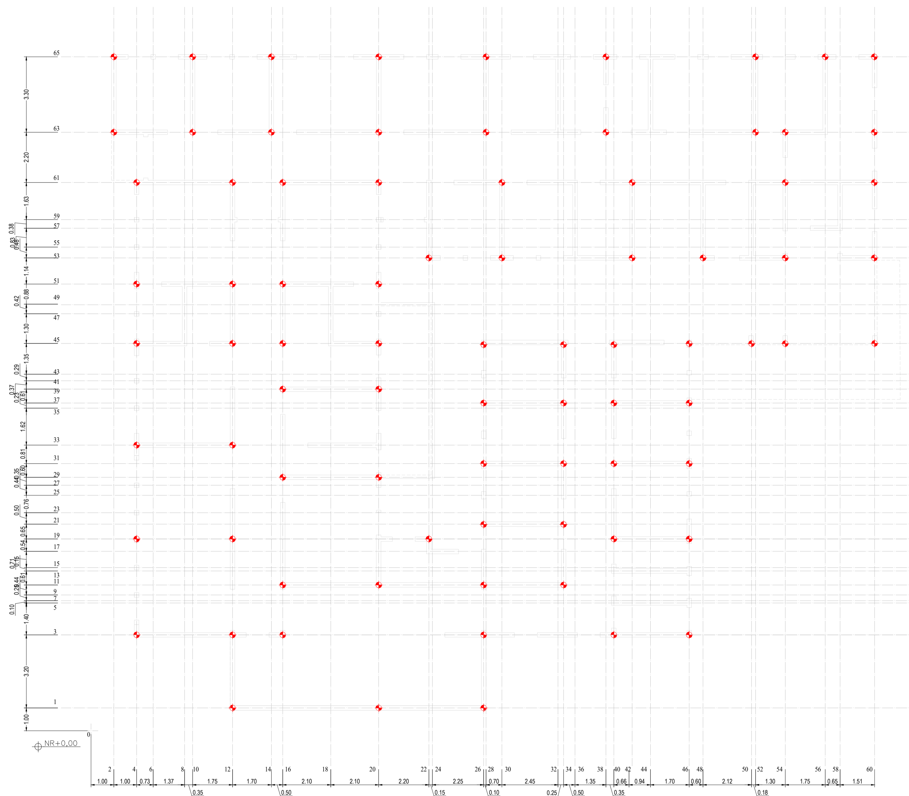
ESTAQUEAMENTO ESCALA 1:100
