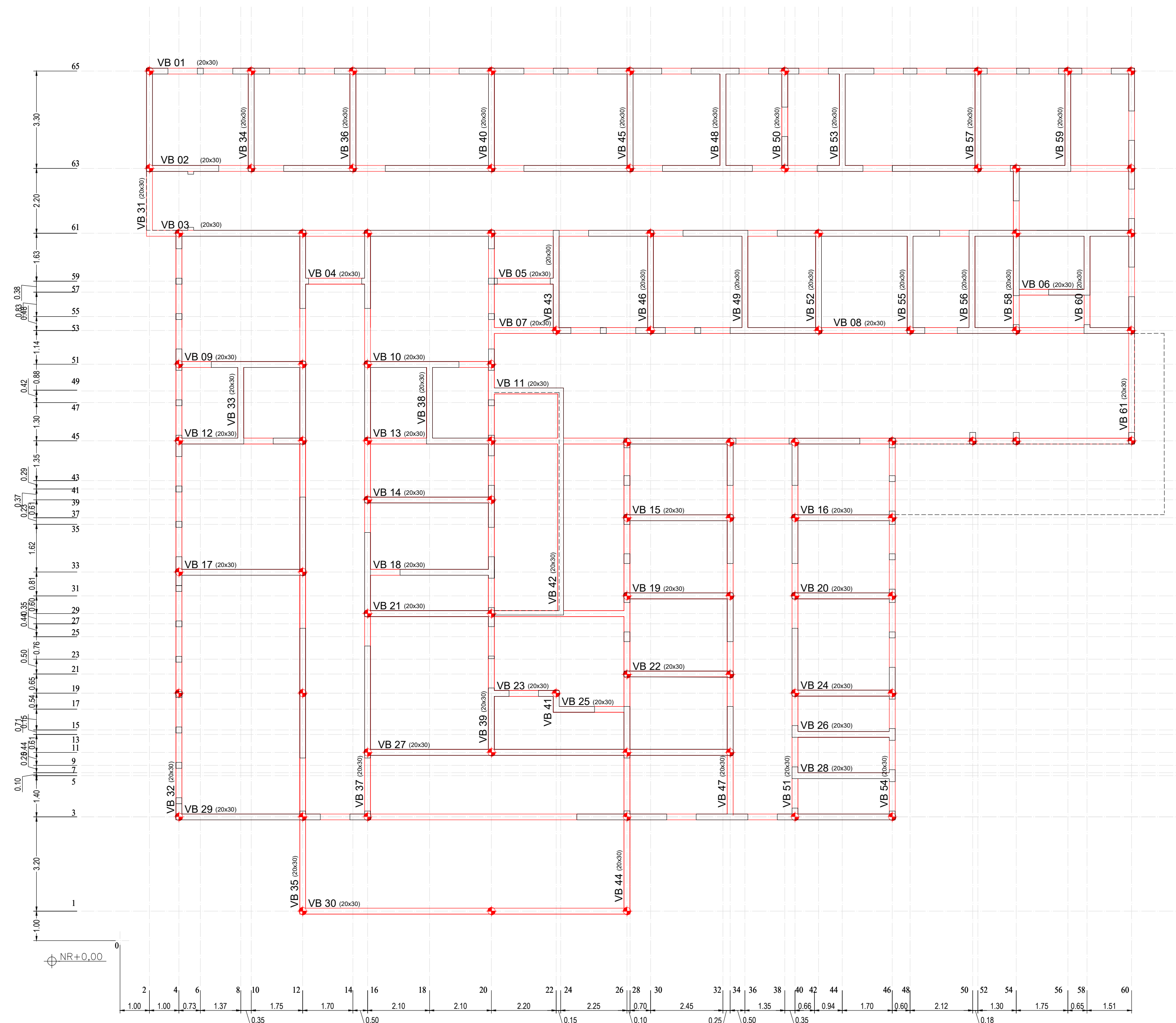
ESQUEMA DE FUNDAMENTAÇÃO ESCALA 1:100
