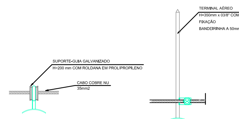
DETALHE 02
