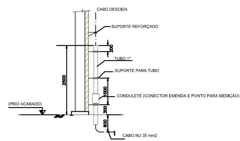
DETALHE DO CONDUTOR DE DESCIDA
