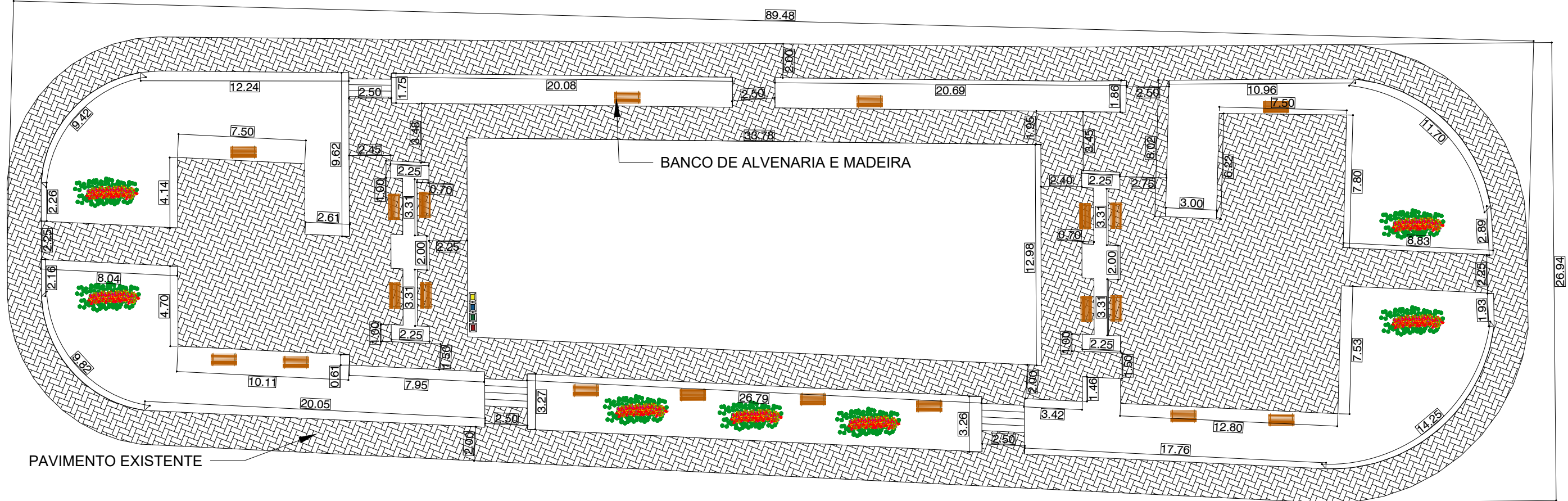
PLANTA BAIXA sem escala
