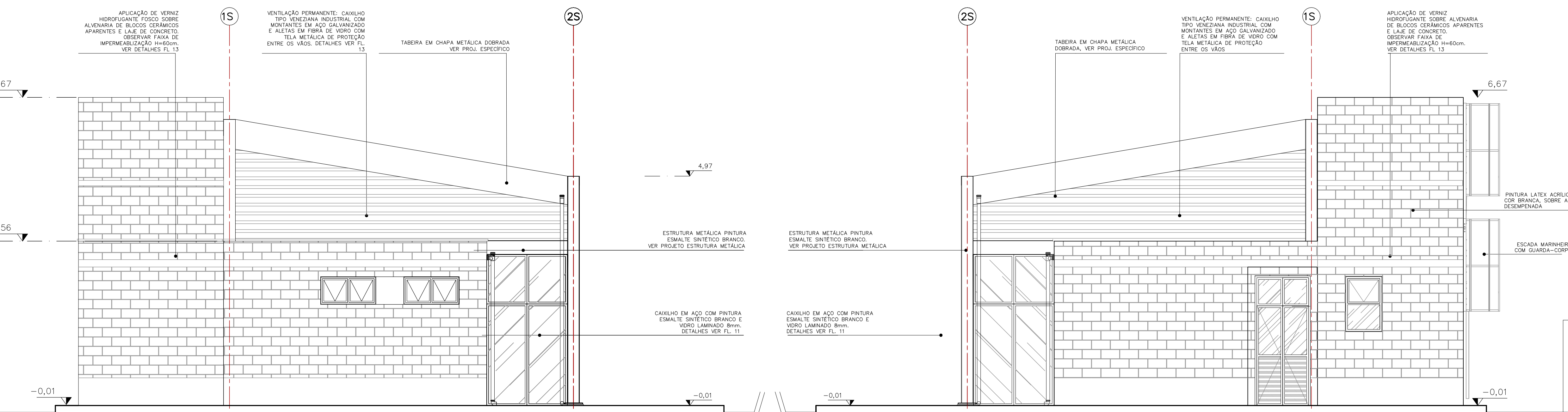
ELEVAÇÃO 2 ESCALA 1:50
