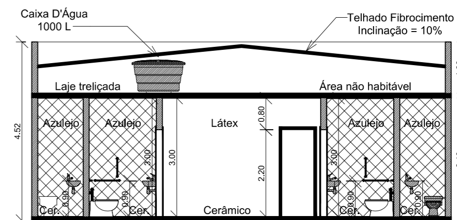
5 Corte B 1 : 100
