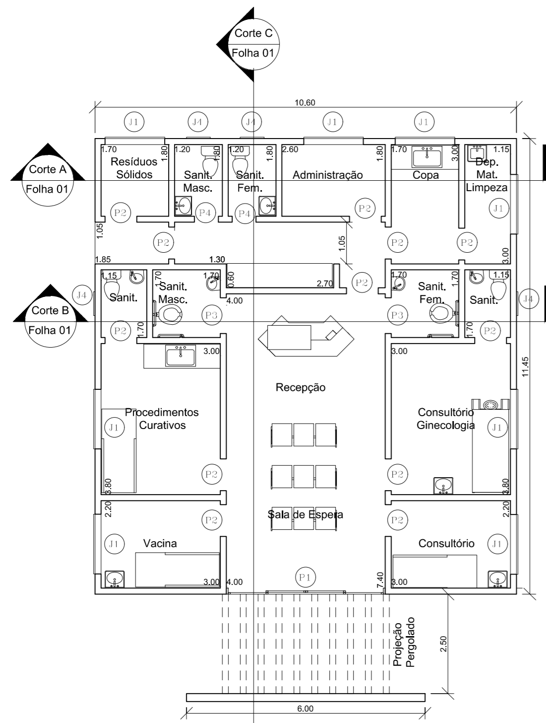
1 Planta 1 : 100
