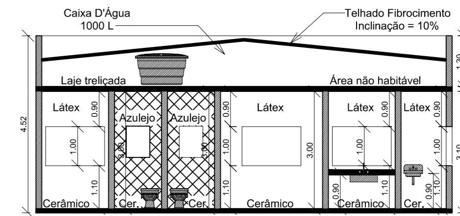
4 Corte A 1 : 100
