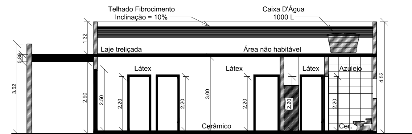
6 Corte C 1 : 100
