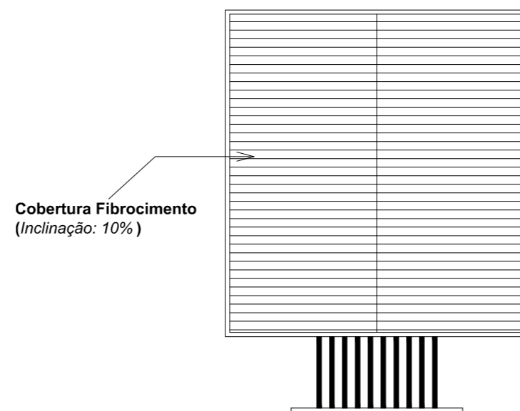
3 Planta Cobertura 1 : 200
