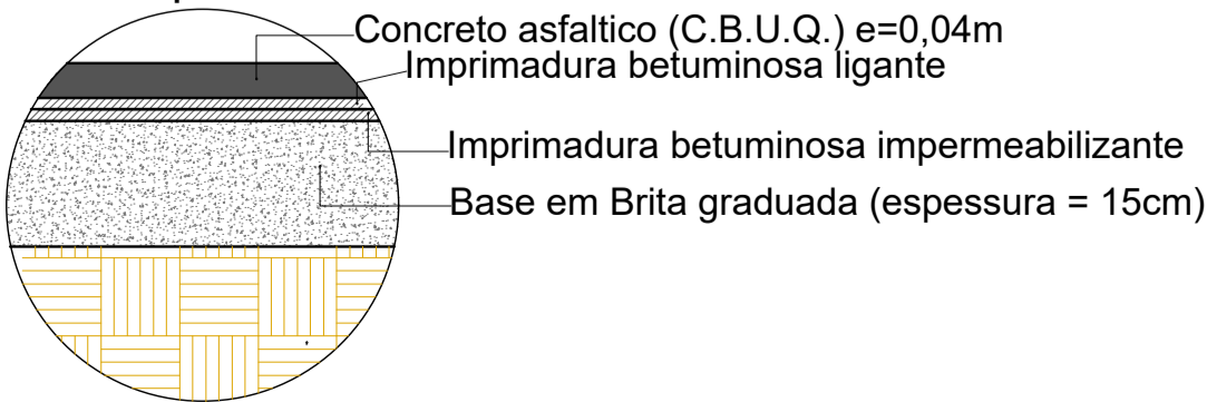
Detalhe 1 (Seção do Pavimento - sem escala) 2ª etapa
