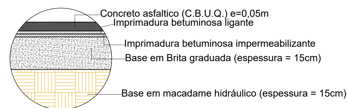
Detalhe 1 (Seção do Pavimento - sem escala)
