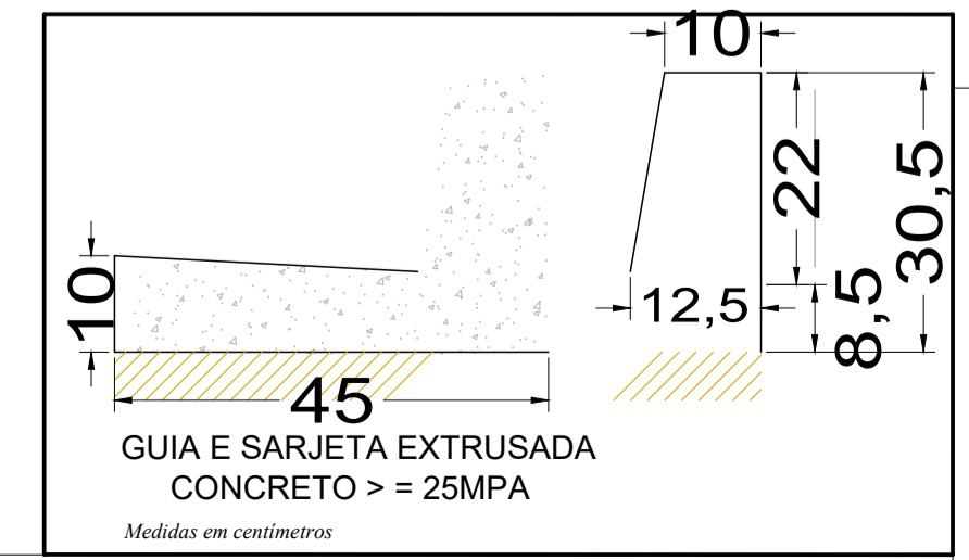
Detalhe 2 (Guia e sarjeta) sem escala
