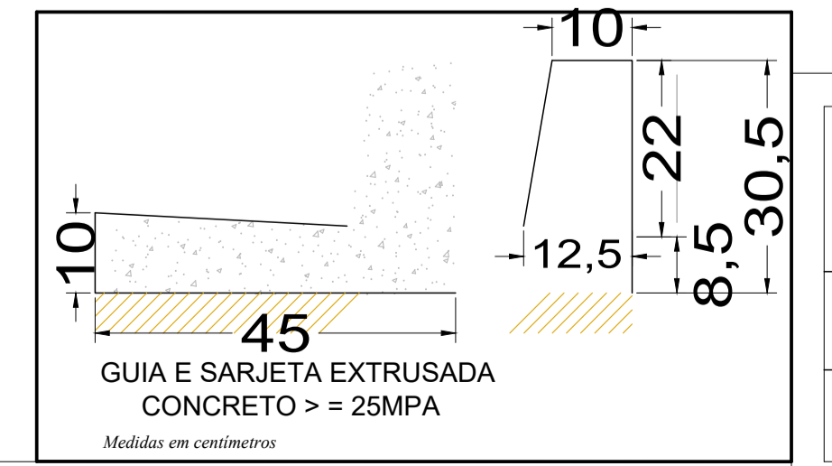
Detalhe 2 (Guia e sarjeta) sem escala
