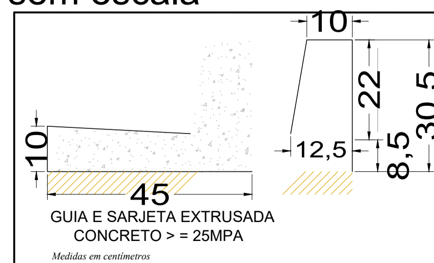
Detalhe 2 (Guia e sarjeta) sem escala
