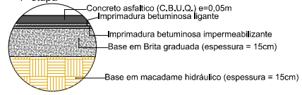
Detalhe 1 (Seção do Pavimento - sem escala) 1ª etapa
