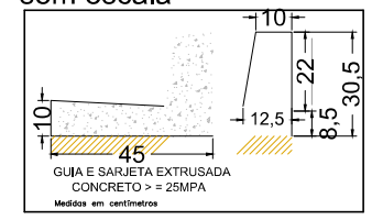
Detalhe 2 (Guia e sarjeta) sem escala
