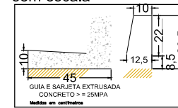
Detalhe 2 (Guia e sarjeta) sem escala
