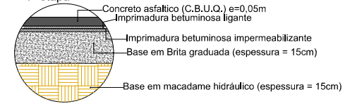
Detalhe 1 (Seção do Pavimento - sem escala) 1ª etapa
